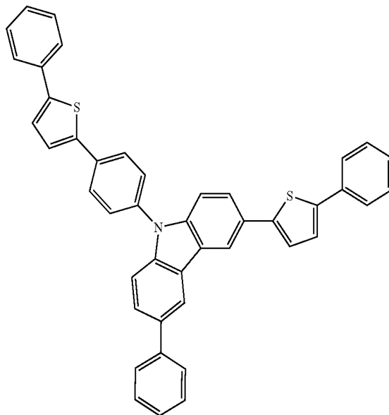
[Formula 5]
